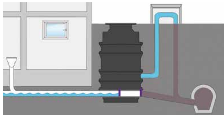
Funktionsdarstellung der Hybrid-Hebeanlage bei Rückstau
