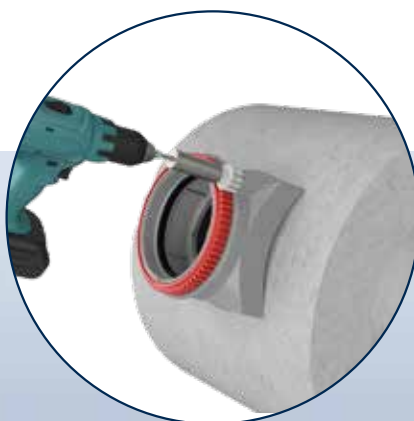
VPS TURBO auf Betonrohr
